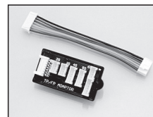
バランス変換ボード (Multiplex, TP, FPタイプ) #44152 ¥630(税込)
